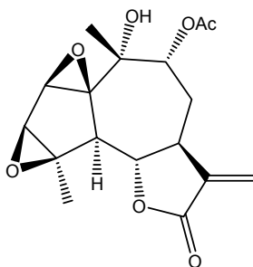
9 \alpha -acetoxartyecanin XVII
